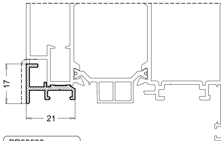
PR58538 0.206 Kg/m
