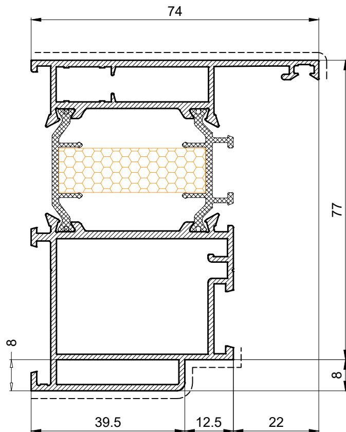
PE85206 1.967 Kg/m
