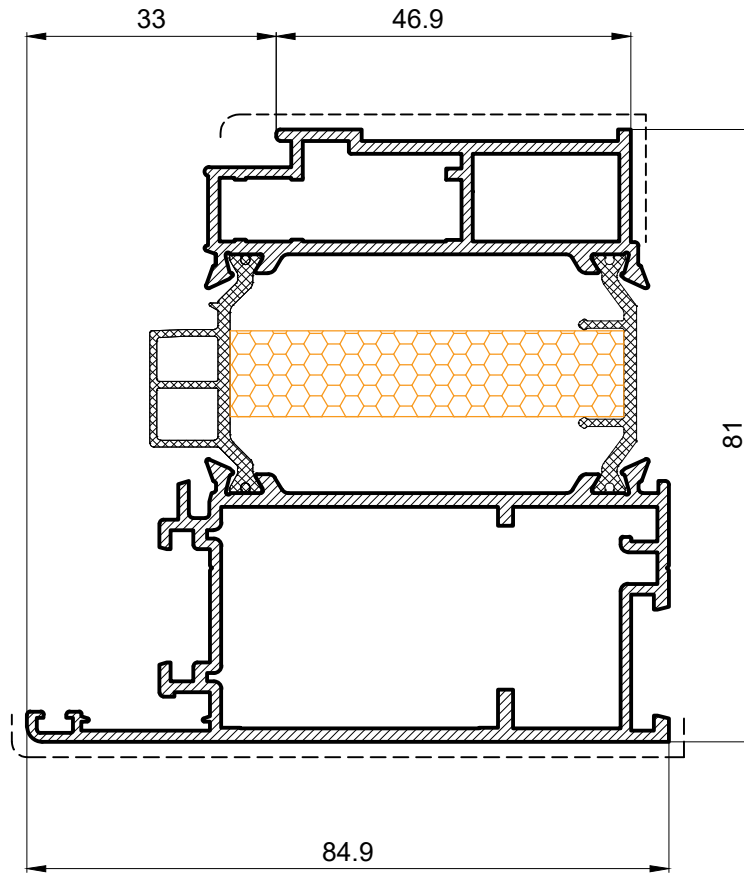
PE85242 2.195 Kg/m
